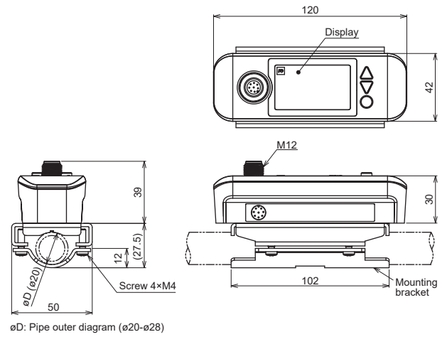
Type: FSZ15
