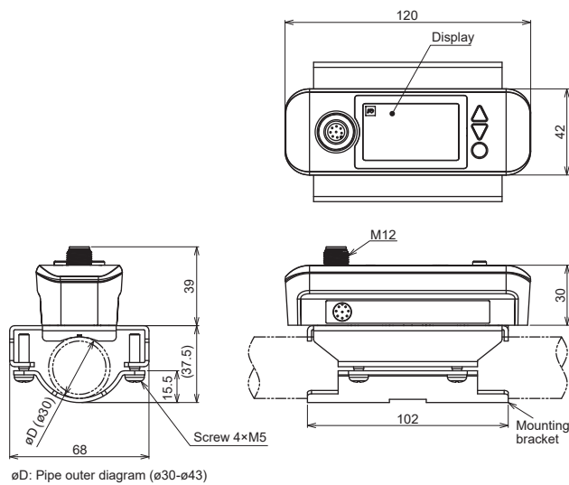
Type: FSZ25
